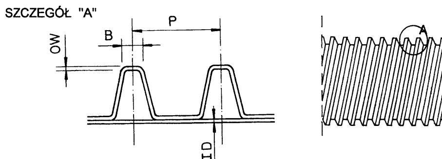
Rys. 2. Przykład złączki zaciskowej do połączenia dwóch rur
