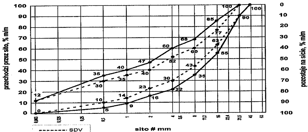
Rysunek 1. Krzywe graniczne uziarnienia mieszanki kruszywa 0/31,5 mm do warstw podbudowy pomocniczej
