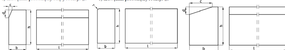
Rysunek 2. Wymiarowanie krawężników
