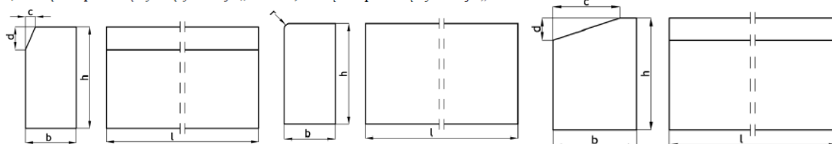
Rysunek 2. Wymiarowanie krawężników
