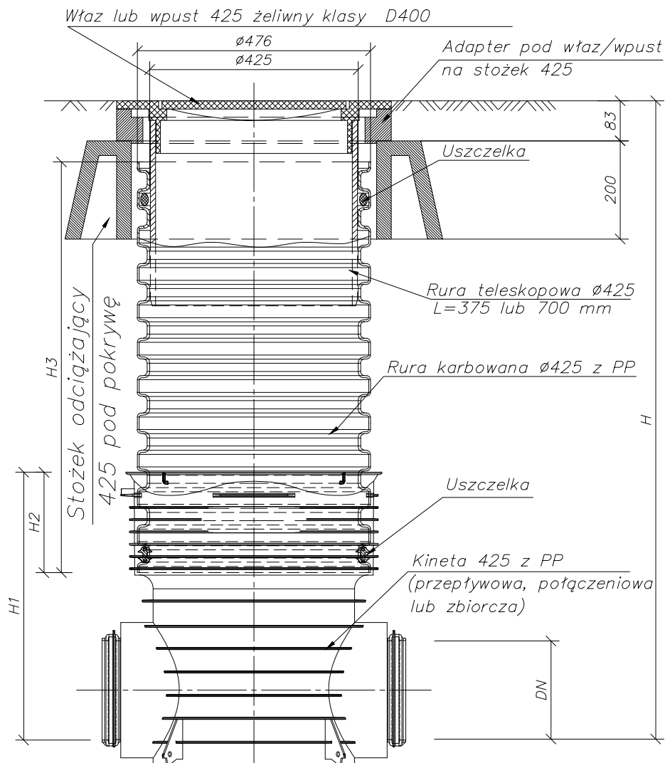
Studzienka inspekcyjna 425 z rurą teleskopową i włazem żeliwnym lub wpustem klasy D na stożku odciągającym 425
