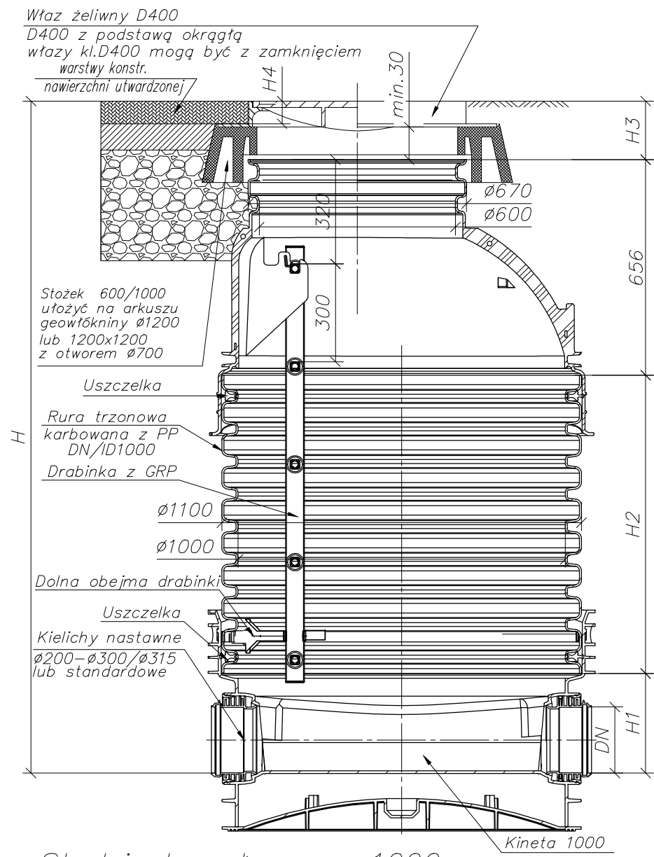
Studzienka włazowa 1000 z włazem klasy D400 na stożku odciążającym
